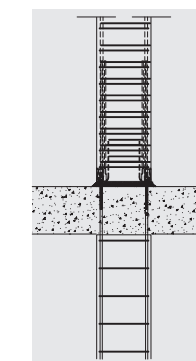
Connessione tipo 2 – Connection type 2
