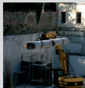
2. Movimentazioni del pilastro – Moving column
